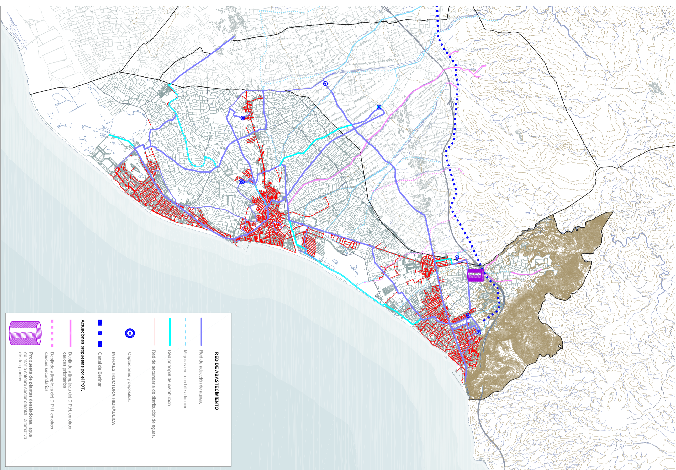
RED DE ABASTECIMIENTO. FUENTE: PLAN DE ORDENACION DEL TERRITORIO DEL PONENTE ALMERIENSE.
