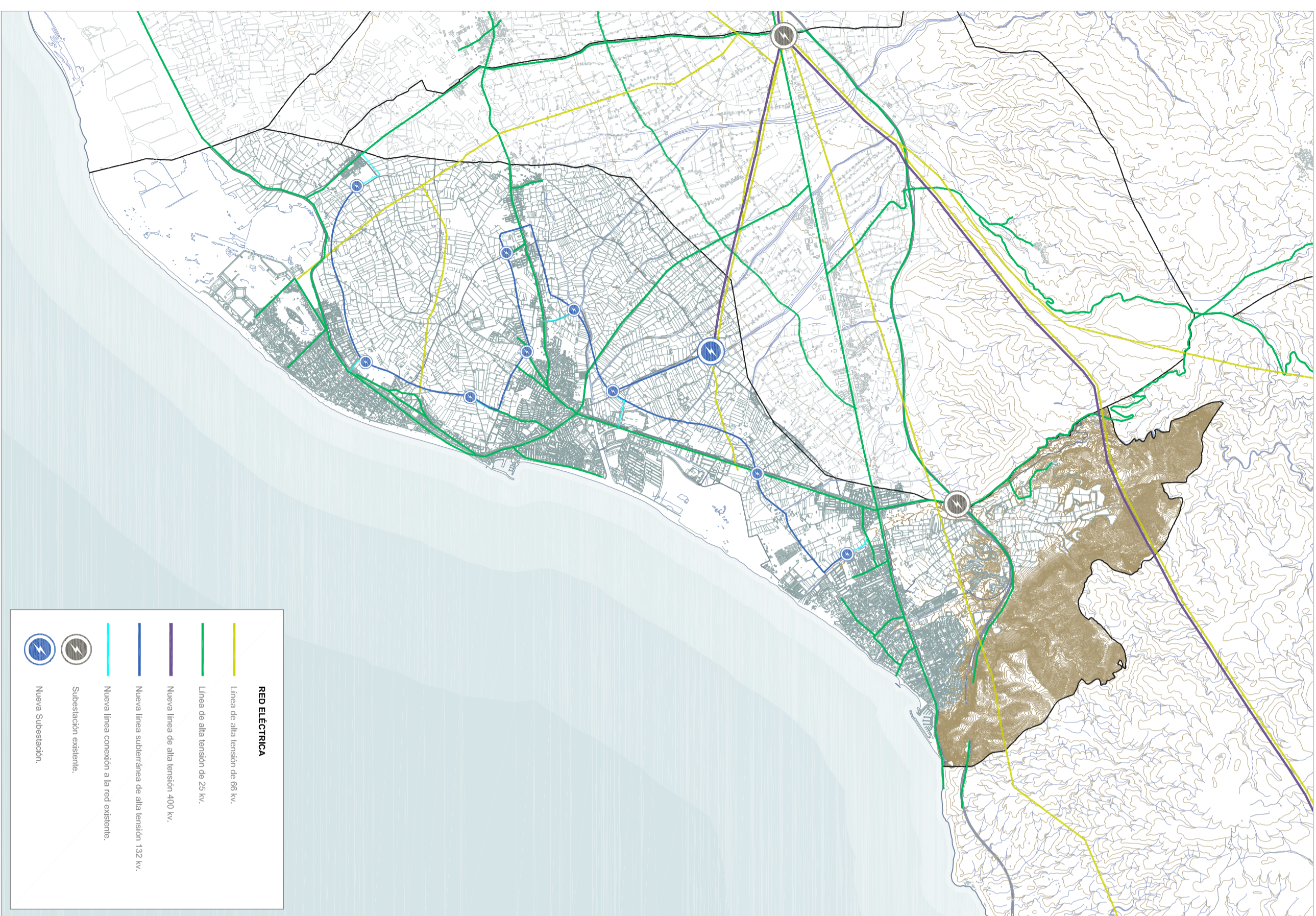
RED DE ENERGIA ELECTRICA. FUENTE: PLAN DE ORDENACION DEL TERRITORIO DEL PONENTE ALMERIENSE.
